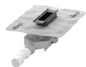
Modell: 4981.81 Ablaufkörper Sanierung Aufbauhöhe: ab 70 mm Sperrwasserhöhe: 25 mm Ablaufleistung: 0,4–0,55 l/s*
