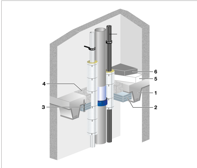
Abb. 151: Stahlbeton- und Spannbeton-Rippendecken bzw. Plattenbalkendecken aus Normalbeton bzw. Leichtbeton mit geschlossenem Gefüge nach DIN 4219-1 und -2 ohne Zwischenbauteile – F 30-, F 60-, F 90-Konstruktion
