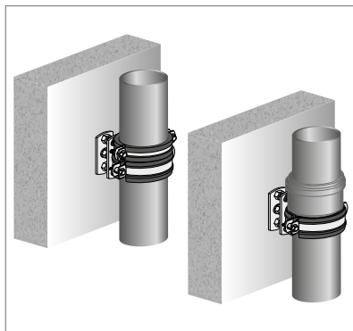
Abb. 259: Rohrschelle mit Entsorgungsleitungen – Beispiele: Festpunkte
