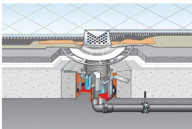
Abb. 237: Rohr-in-Rohr-Technik für Bodenablauf
