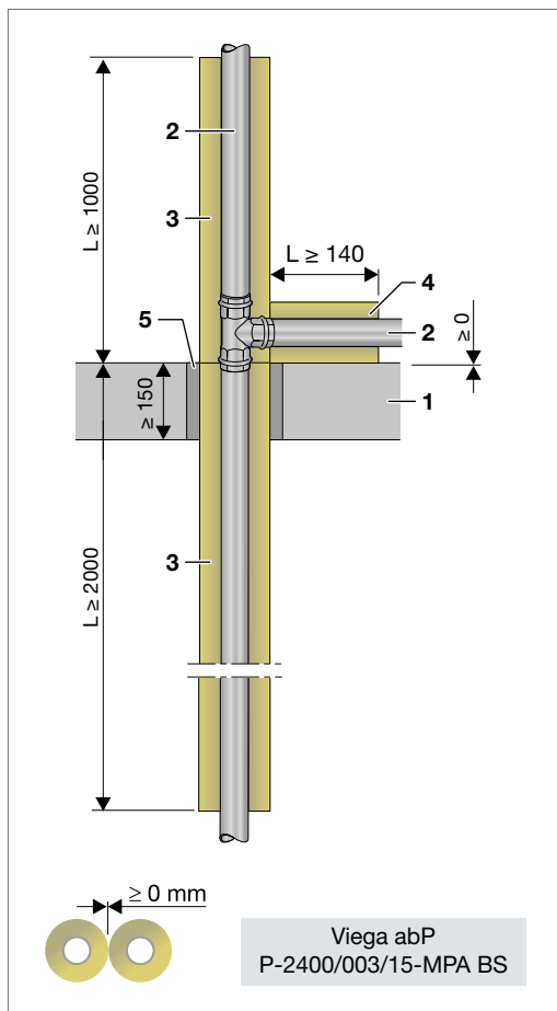
Abb. 92: Etagenanzug mit Prestabo/Prestabo PP-ummantelt – oberhalb der Decke
