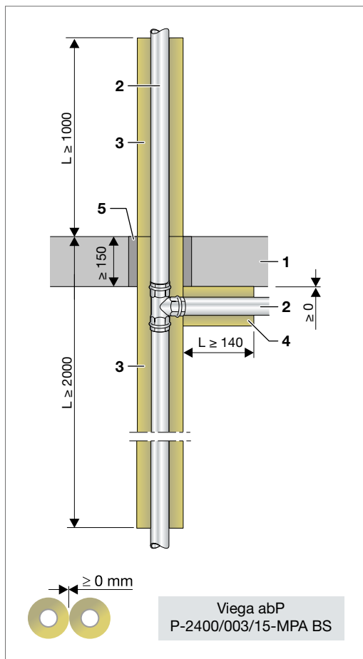
Abb. 82: Etagenansbindung mit Temponox – unterhalb der Decke
