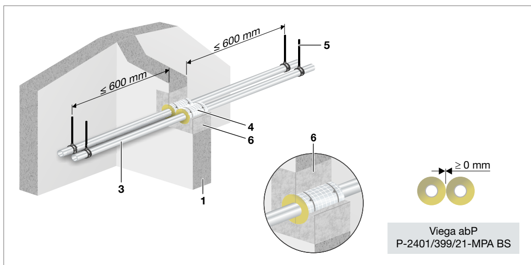
Abb. 171: Raxinox – Einbau in Massivwand
