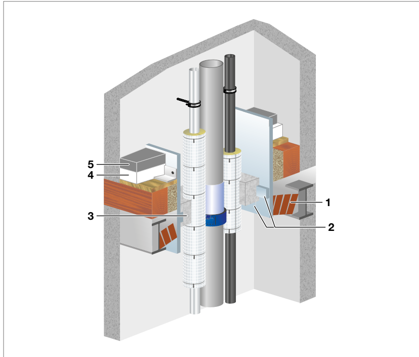
Abb. 153: Gewölbedecke mit Mörtelverguss – F 30-, F 60-, F 90-Konstruktion
