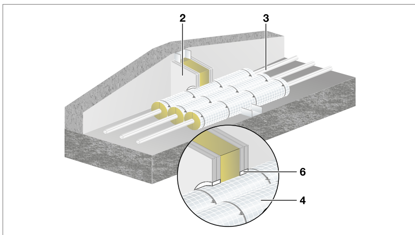
Abb. 193: Wandschließung mit Sanfix Fosta/Raxofix durch leichte Trennwand, R 30/R 60/R 90
