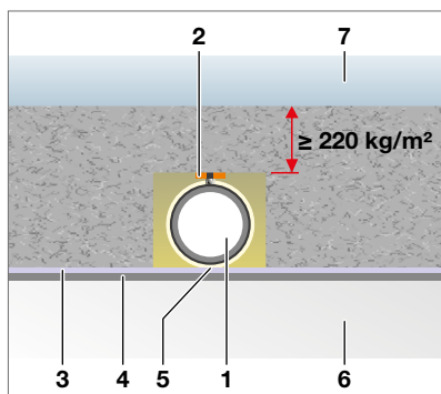
Abb. 277: Körperschallentkopplung in der Wand
