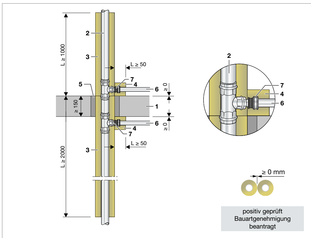
Abb. 32: Etagenanschlüsse mit Viega Metallrohrsystem und Übergang auf Raxinox
