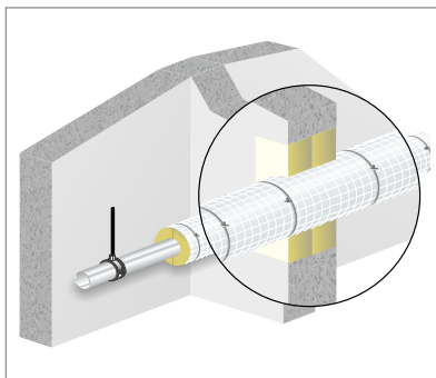
Abb. 204: Dämmung durch Weichschott hindurchgeführt – Wand
