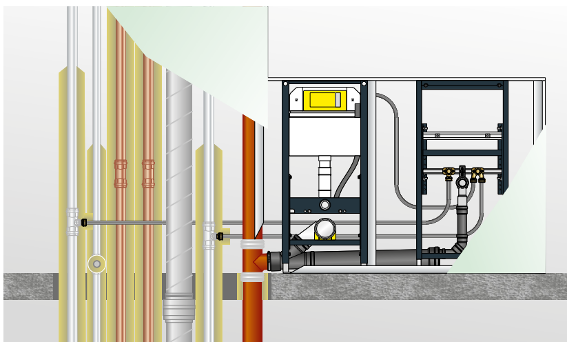
Abb. 54: Wirtschaftlicher Schachtaufbau mit Guss SML Fallleitung
