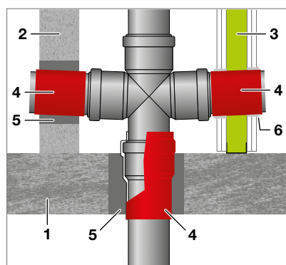
Abb. 276: Körperschallentkopplung
