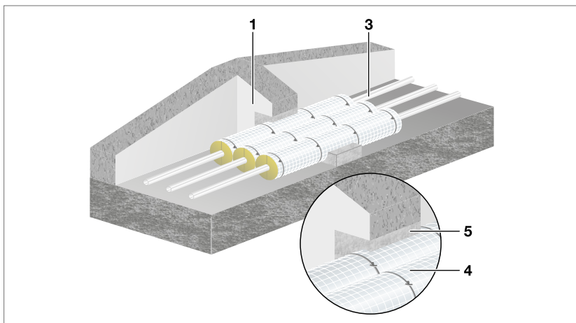
Abb. 192: Wandschließung mit Sanfix Fosta/Raxofix durch Massivwand, R 30/R 60/R 90
