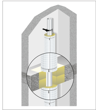
Abb. 203: Unterbrochene Dämmung – Decke
