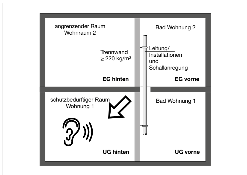
Abb. 254: Schnittzeichnung des Installationsprüfstands im Fraunhofer-Institut für Bauphysik. Der Prüfstand besteht aus je zwei übereinanderliegenden Räumen im Erd- und Untergeschoss (EG und UG), sodass in Verbindung mit Dach- und Kellergeschoss (DG und KG) auch über mehrere Stockwerke reichende Installationen, wie z. B. Abwassersysteme, geprüft werden können.
