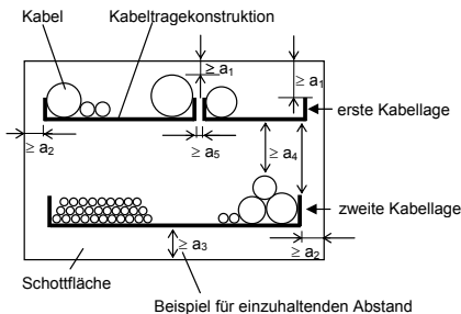
Beispiel D: Abstand zwischen "Kabellagen"; Ansicht
