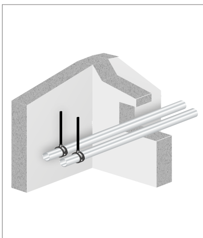
Abb. 257: Rohrschelle mit Versorgungsleitungen - Einbausituation Wand
