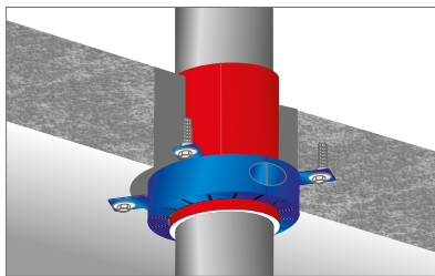
Abb. 263: Montagebeispiele von Brandschutzmanschette mit Schallschutzmatte aus PE, s = 5 mm (aufgesetzt)
