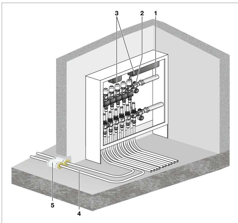
Abb. 189: Rohrdurchführungen R 30/R 60/R 90
