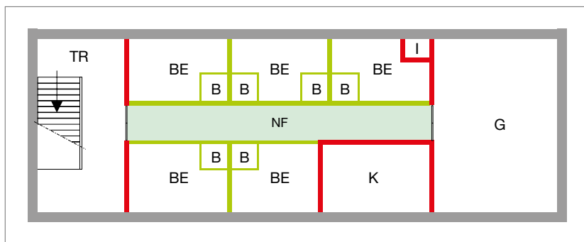
Abb. 215: Trennwände Beherbergungsstättenverordnung — MBeVO
