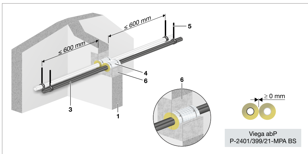
Abb. 169: Raxofix/Sanfix Fosta, d \leq 16 \text{ mm} – Einbau in Massivwand
