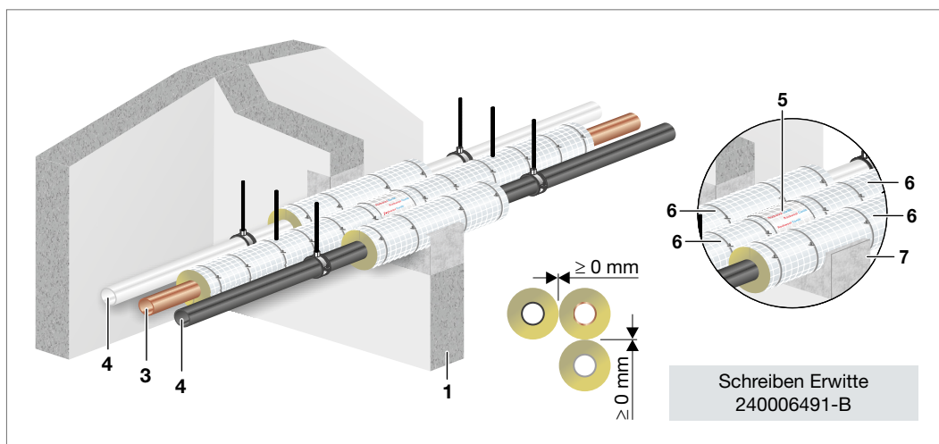
Abb. 177: Viega Kunststoffrohrsysteme im Nullabstand Rockwool Conlit 150U abP P-3725/4130-MPA-BS – Massivwand
