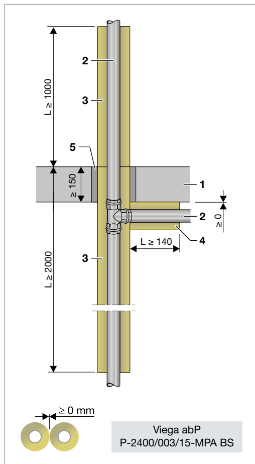
Abb. 93: Etagenanzug mit Prestabo/Prestabo PP-ummantelt – unterhalb der Decke
