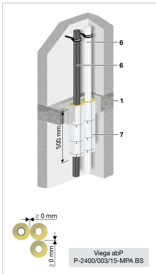
Abb. 117: Nullabstand Viega Rohrleitungssysteme Raxofix zu Sanfix Fosta
