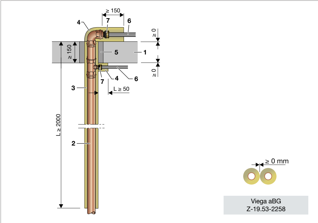
Abb. 67: Etagenanzubindung/oberstes Geschoss mit Profipress und Übergang auf Raxofix/Sanfix Fosta
