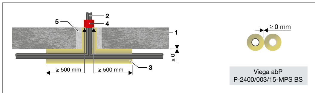
Abb. 109: Raxofix/Sanfix Fosta mit Rockwool 800
