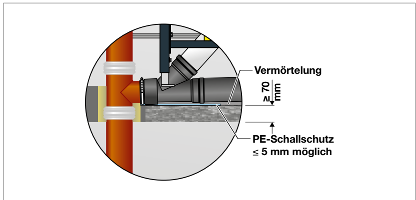
Abb. 49: Detail/Tiefer Einbau
