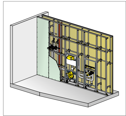
Abb. 291: Prevista Dry Plus – Inwandmontage
