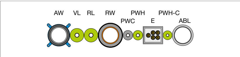
Abb. 201: optimierter Schacht durch Viega Brandschutzsystem mit Regenwasserleitung im Schacht
