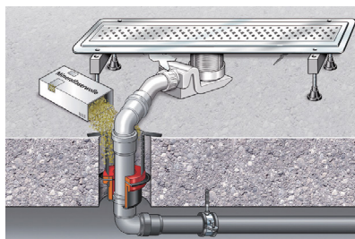
Abb. 238: Rohrdurchführung bei Advantix-Duschrinne
