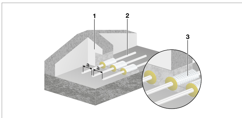
Abb. 195: Wanddurchführung Fonterra Rohre/Raxofix/Sanfix Fosta nach LAR
