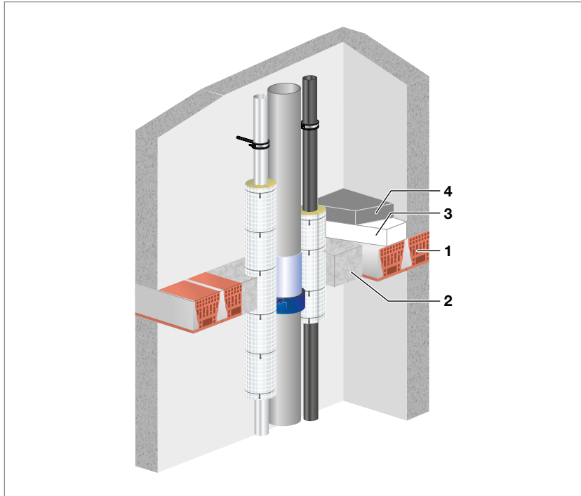
Abb. 149: Stahlbeton- und Spannbeton-, Balken- und Rippendecken aus Normalbeton mit Zwischenbauteilen F 90-Konstruktion
