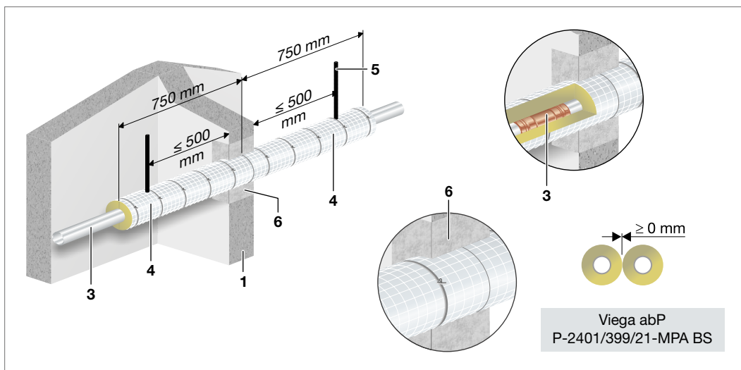
Abb. 161: Temponox in Verbindung mit Profipress Verbindern – Einbau in Massivwand
