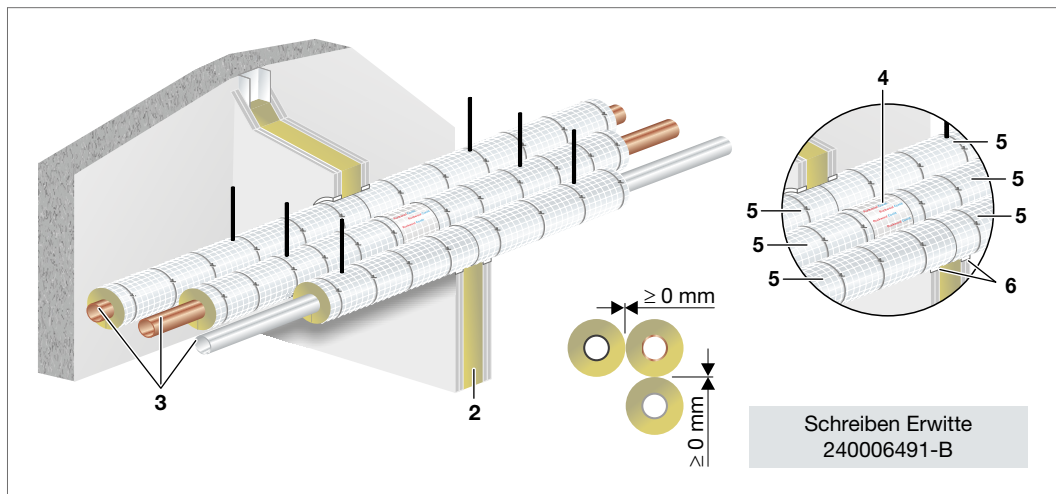
Abb. 176: Viega Metallrohrsysteme im Nullabstand Rockwool Conlit 150U ab P-3725/4130-MPA-BS – leichte Trennwand
