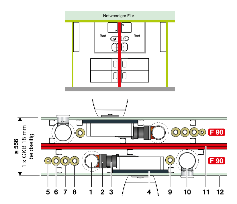
Abb. 229: F 90 Leichte Trennwand mit beidseitiger Wandbelegung
