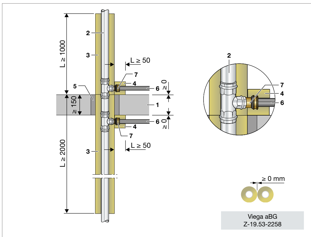
Abb. 27: Etagenanbindung mit Viega Metallrohrsystem und Übergang auf Raxofix/Sanfix Fosta
