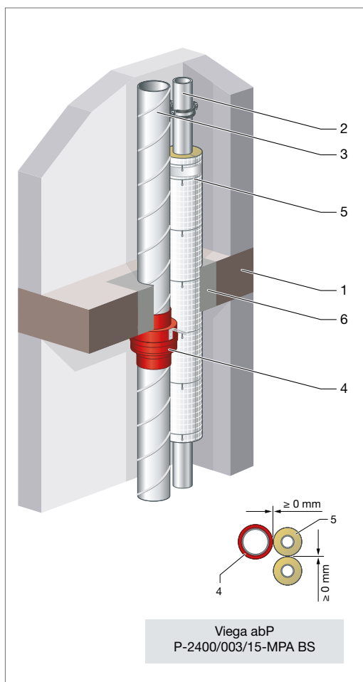
Abb. 142: 0-Abstand zu Absperrvorrichtungen K 90-18017-3 (Bartholomäus AVR/Wildeboer TS 18)
