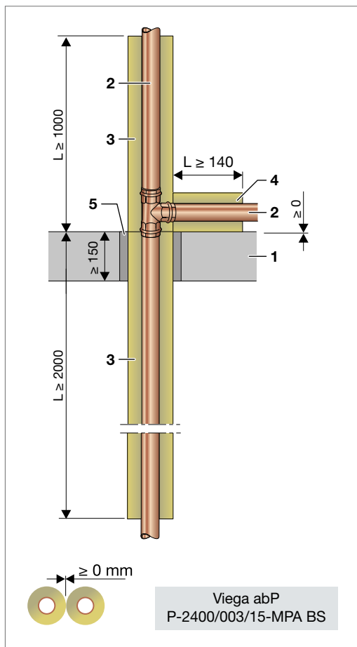
Abb. 65: Etagenbindung mit Profipress – oberhalb der Decke
