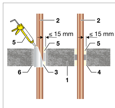
Abb. 197: Viega Brandschutz-Kitt-Abschottung mit Hüllrohr oder in Kernbohrung
