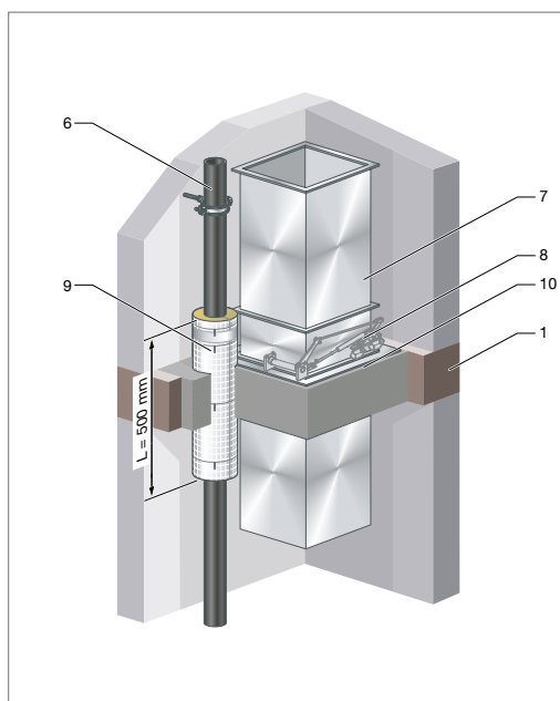
Abb. 145: Brandschutzklappen/EN1366-2
