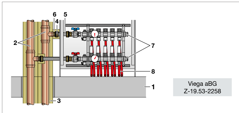
Abb. 184: Fußbodenheizung mit Viega Bauartgenehmigung
