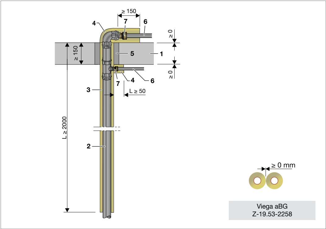
Abb. 104: Etagenansbindung/oberstes Geschoss mit Megapress und Übergang auf Raxofix/Sanfix Fosta
