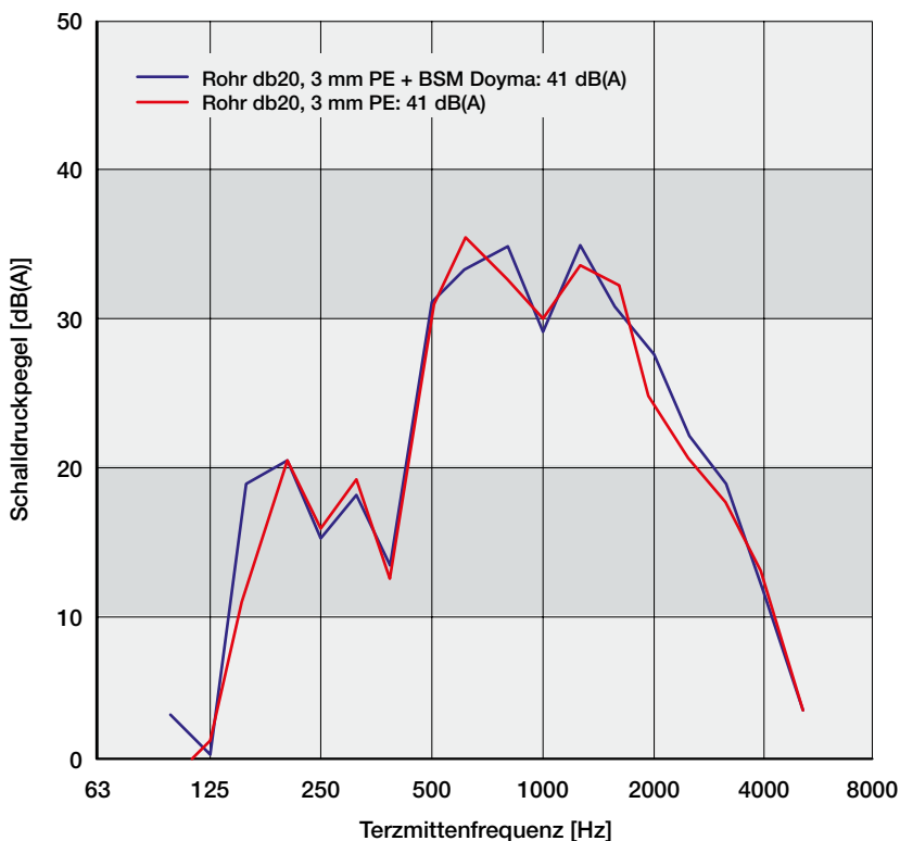
Abb. 267: Summenschallpegel im UG hinten
