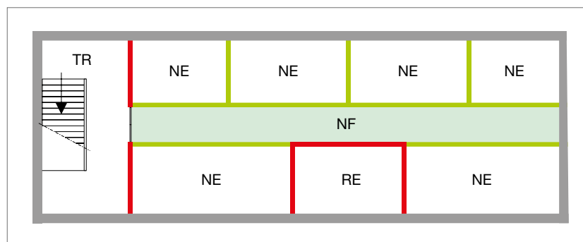
Abb. 185: Notwendiger Flur und Trennwände nach Musterbauordnung — MBO
