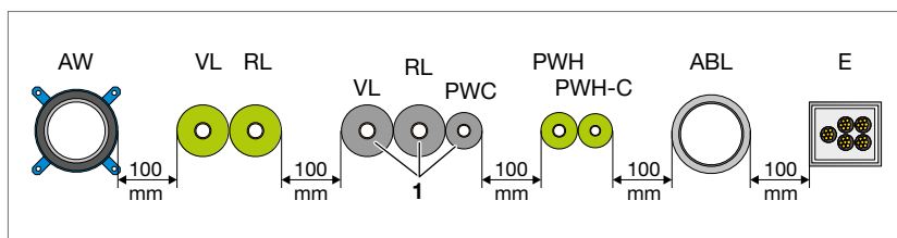
Abb. 198: Schachtbelegung unter Einhaltung der Abstandsregeln
