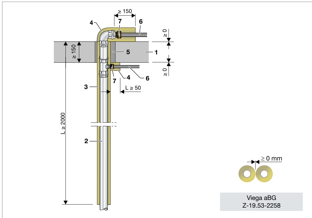
Abb. 77: Etagenankbindung/oberstes Geschoss mit Sanpress/Sanpress Inox und Übergang auf Raxofix/Sanfix Fosta
