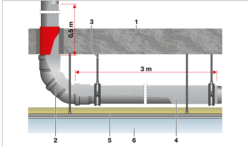
Abb. 278: Ummantelung mit Bleifolie zur Schalldämmung
