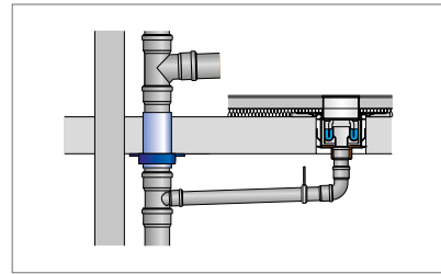
Abb. 231: Viega Advantix R 120 Bodenablauf und Rohrdurchführung – brennbare Entwässerungsleitungen
