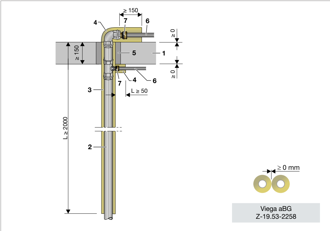
Abb. 94: Etagenanbindung/oberstes Geschoss mit Prestabo und Übergang auf Raxofix/Sanfix Fosta
