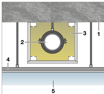
Abb. 279: Einhausung von Entsorgungsleitungen
