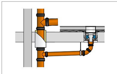
Abb. 232: Viega Advantix R 120 Bodenablauf und Rohrdurchführung – nicht-brennbare Entwässerungsleitungen
