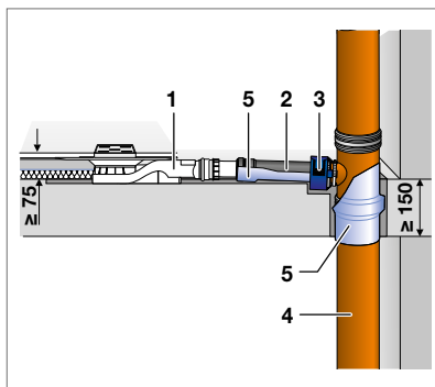
Abb. 245: Viegas Bodenablauf – Mischinstallation
