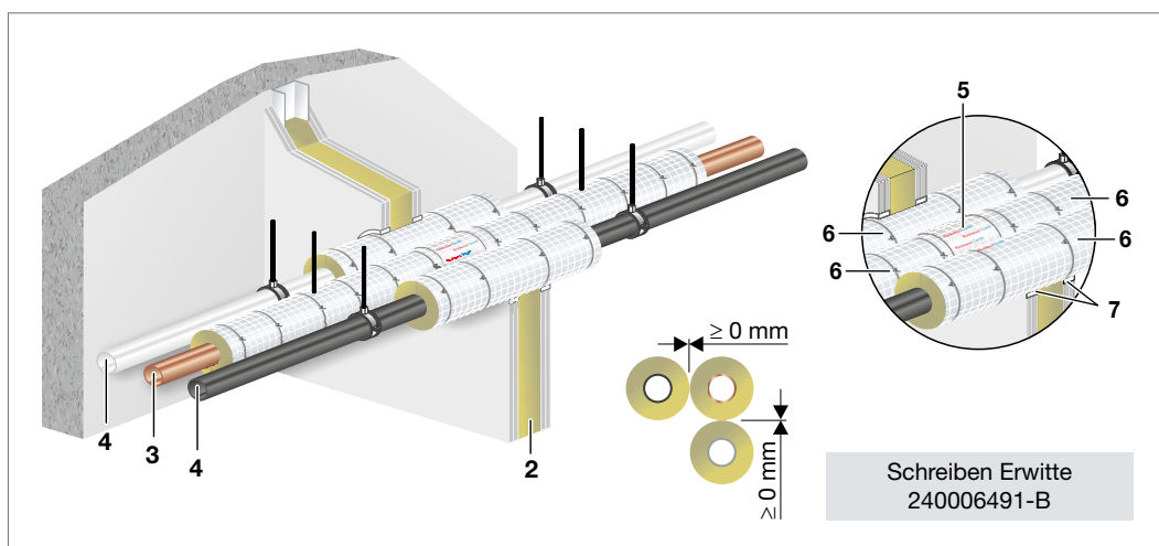
Abb. 178: Viega Kunststoffrohrsysteme im Nullabstand Rockwool Conlit 150U abP P-3725/4130-MPA-BS – leichte Trennwand
