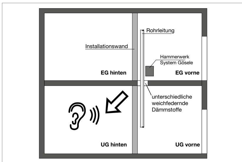
Abb. 255: Schnittzeichnung des Installationsprüfstands im Fraunhofer-Institut für Bauphysik. Der Prüfstand besteht aus je zwei übereinanderliegenden Räumen im Erd- und Untergeschoss (EG und UG), sodass in Verbindung mit Dach- und Kellergeschoss (DG und KG) auch über mehrere Stockwerke reichende Installation, wie z. B. Abwassersysteme, geprüft werden können.
