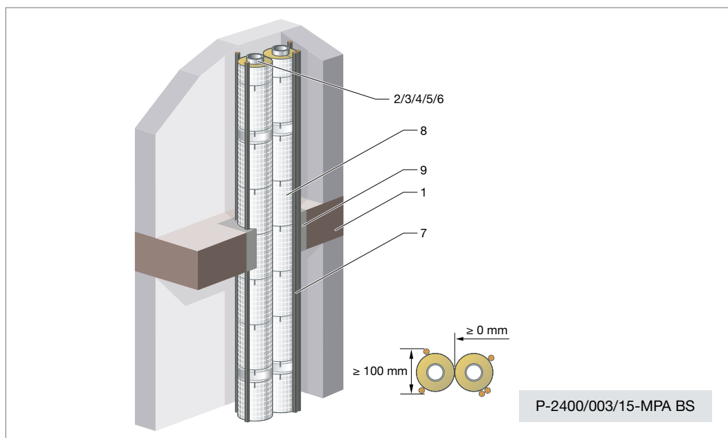
Abb. 146: Einbau und Anordnung von Begleitkabeln
