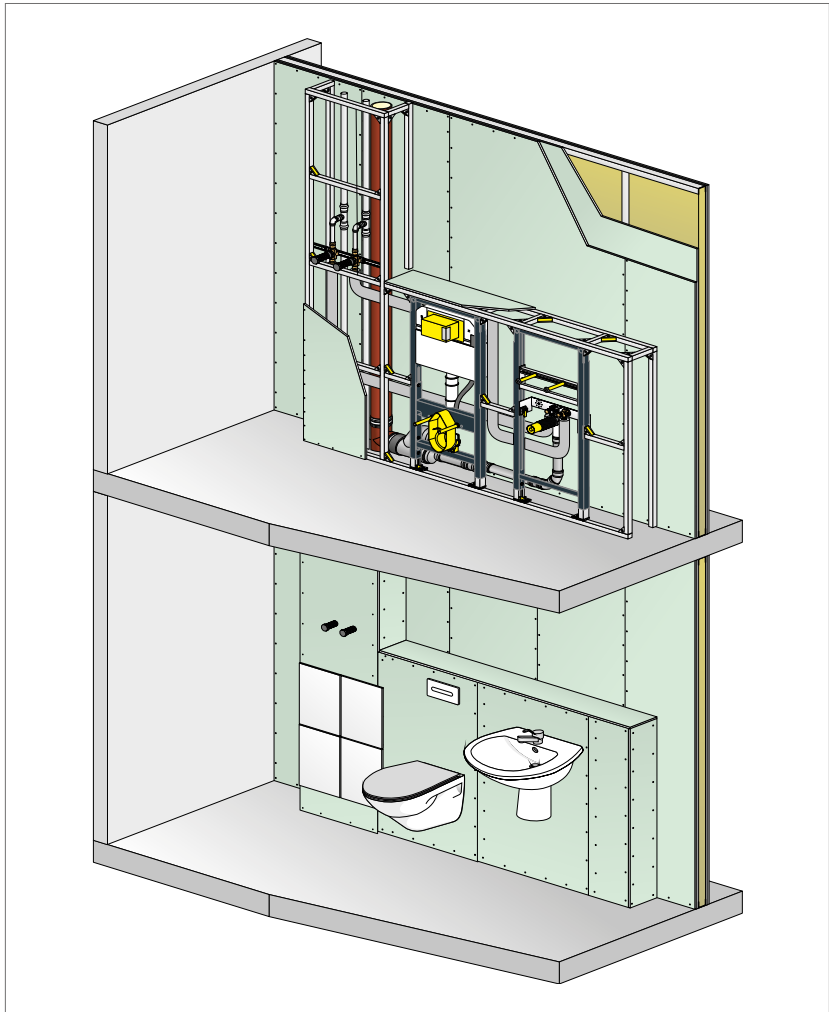
Abb. 296: Vorwand-Installation mit Prevista Dry Plus vor leichter Trennwand (Darstellung beispielhaft)
