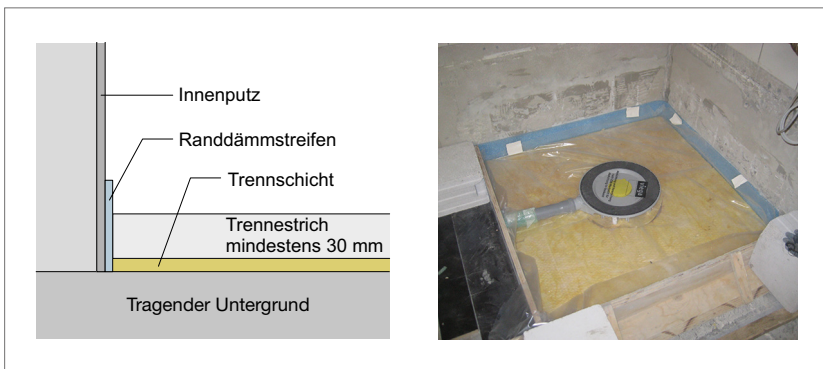
Abb. 289: Der Randdämmstreifen muss lückenlos und vollständig auch hinter dem Bodenablauf durchgeführt werden und dabei großzügig über der Estrich-Oberkante überstehen.
