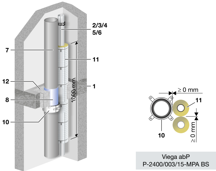
Abb. 130: Beispiel – Brandschutzmanschette Geberit Rohrschott90 Plus nur mit db20, Silent-PP, nach Tab. 53
