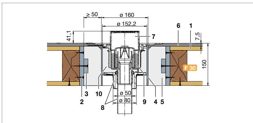
Abb. 242: Beispiel: Viega Brandschutz Advantix-Badablauf mit umlaufender Vermörtelung \geq 50 mm
