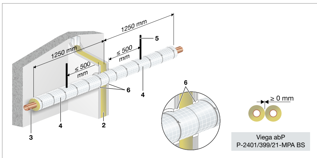
Abb. 156: Profipress/Profipress mit Smartloop Inliner-Zirkulation – Einbau in leichter Trennwand
