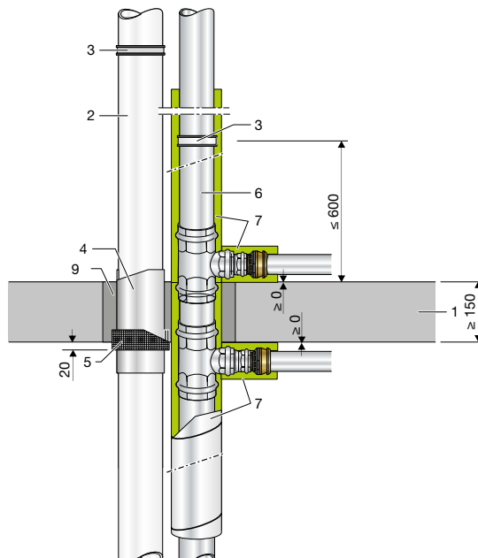
Abb. 136: Abstände zwischen Abschottungen nach dieser abG und Abschottungen nach abG Nr. Z-19.53-2258
