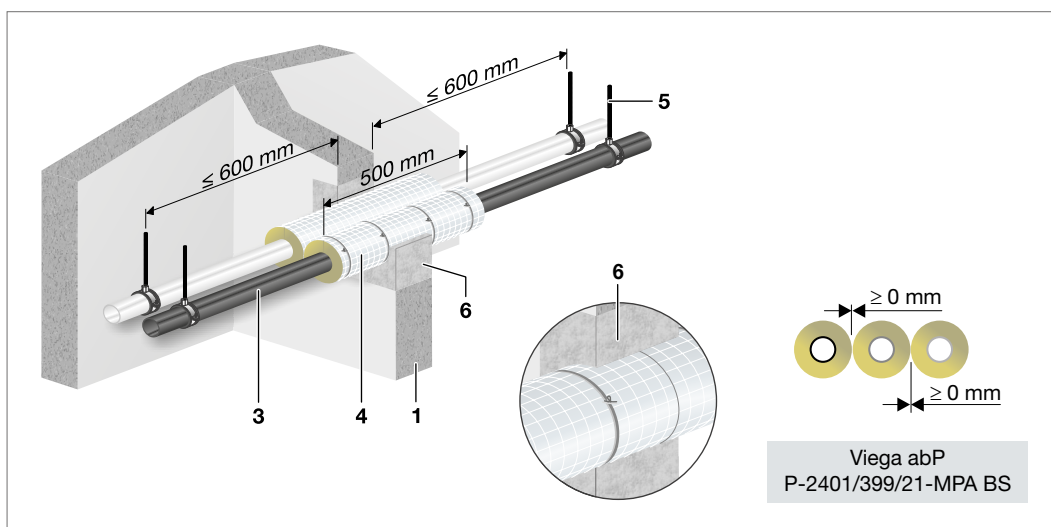
Abb. 167: Raxofix/Sanfix Fosta, d 16 - 63 mm – Einbau in Massivwand
