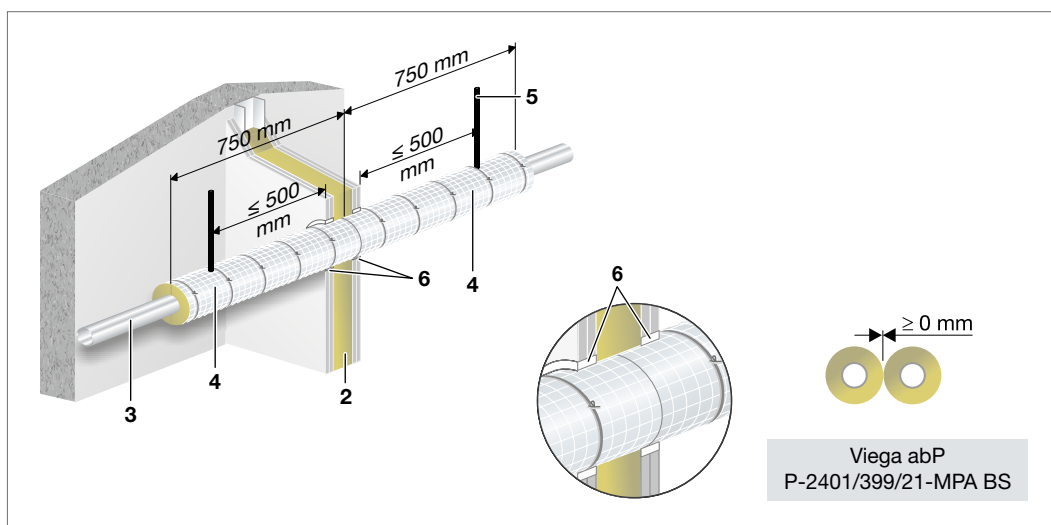
Abb. 160: Temponox – Einbau in leichte Trennwand
