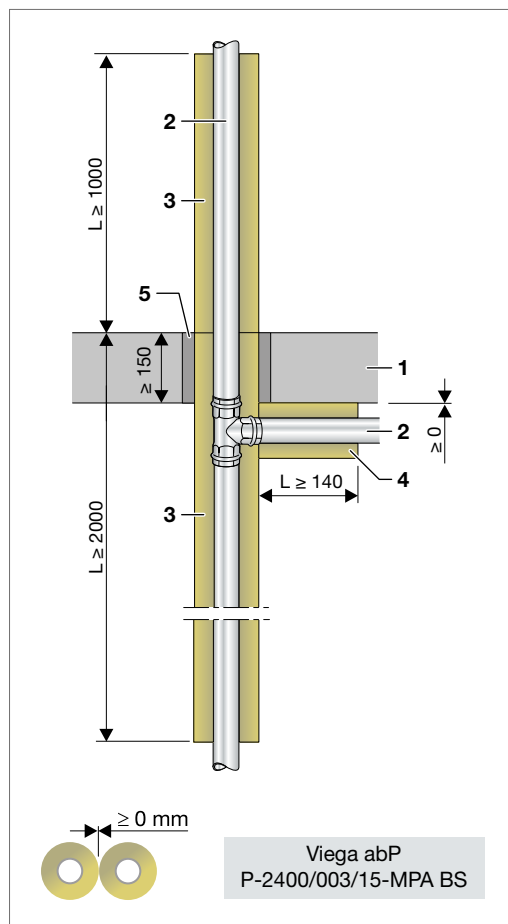
Abb. 76: Etagenansbindung mit Sanpress/Sanpress Inox – unterhalb der Decke
