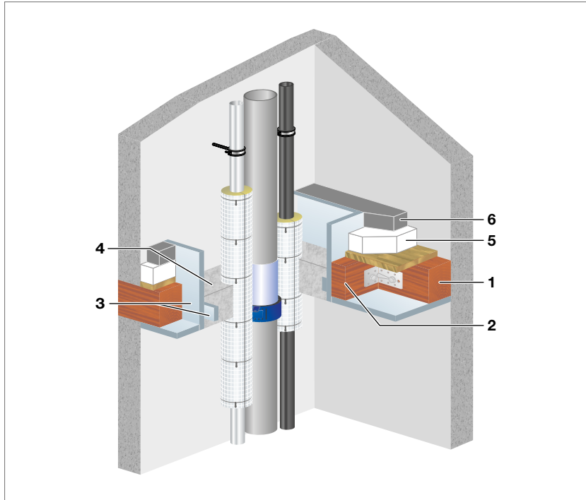
Abb. 147: Holzbalkendecke mit Mörtelverguss F 30-Konstruktion
