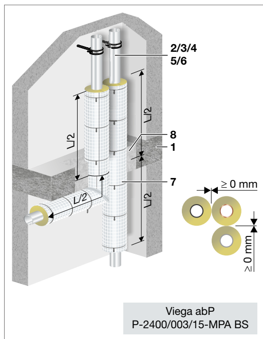
Abb. 118: Einbauvarianten Verzug unterhalb der Decke
