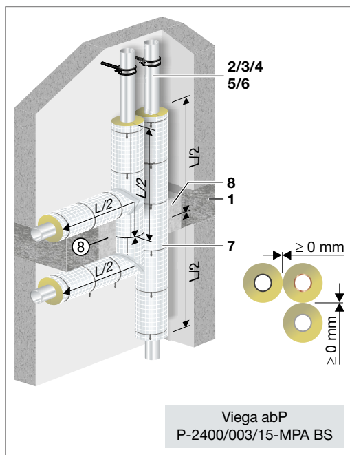
Abb. 119: Einbauvarianten Verzug unter-/oberhalb der Decke
