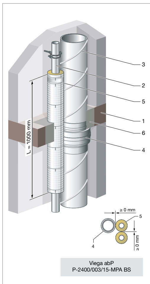
Abb. 143: 0-Abstand zu Absperrvorrichtungen K 90-18017-3 (Bartholomäus AVR/Wildeboer TS 18)
