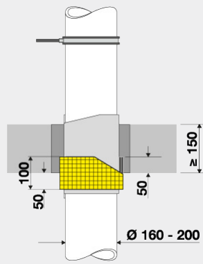
Aufbau Typ 2 (100 mm)
