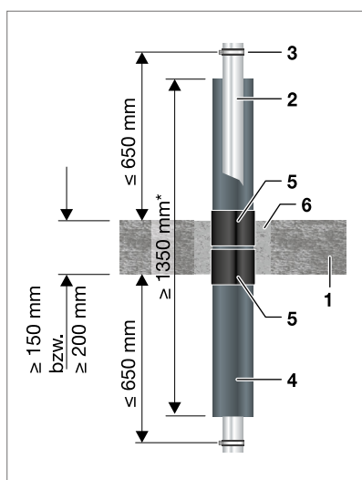
Abb. 199: Brandschutz mit Kaiflex Pyrostar
