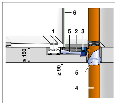
Abb. 246: Viegas Duschrinne – Mischinstallation
