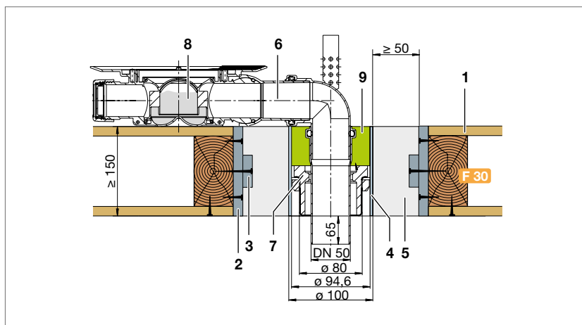
Abb. 244: Beispiel: Viega Advantix-Rohrdurchführung mit umlaufender Vermörtelung \geq 50 mm
