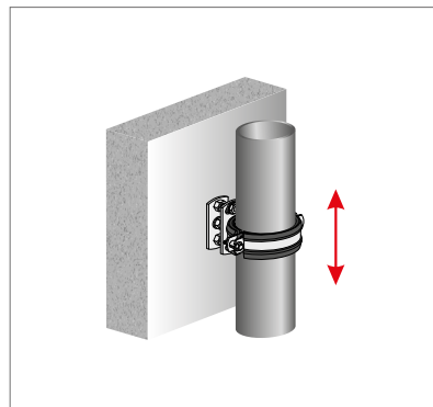
Abb. 260: Rohrschelle mit Entsorgungsleitungen – Beispiel: Gleitschelle
