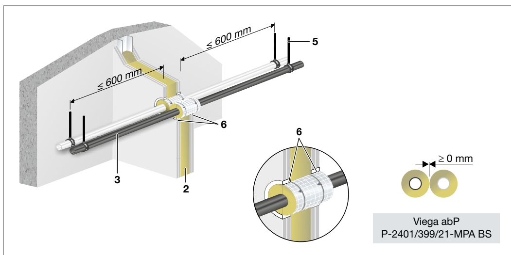
Abb. 170: Raxofix/Sanfix Fosta, d \leq 16 \text{ mm} – Einbau in leichte Trennwand
