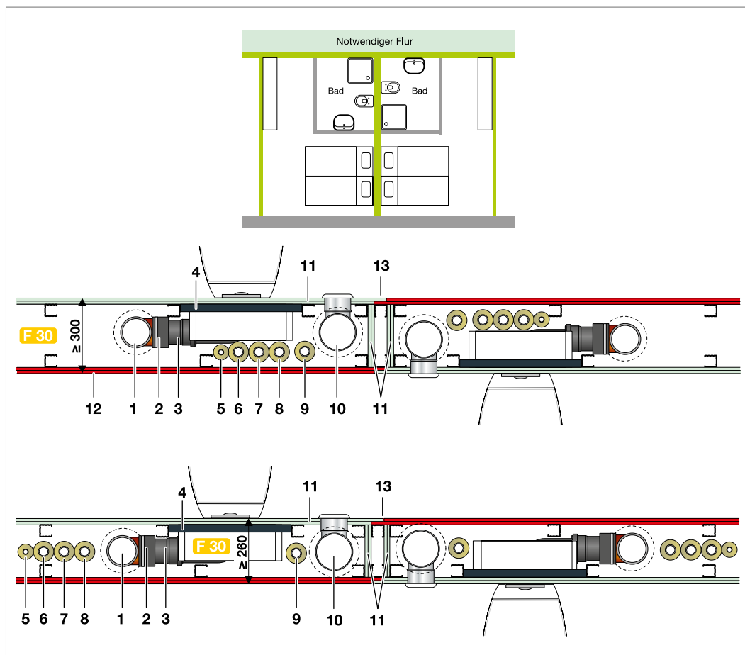
Abb. 226: F 30 Leichte Trennwand mit beidseitiger Wandbelegung
