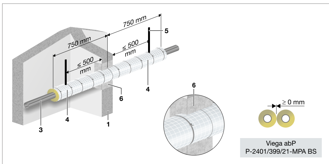
Abb. 165: Megapress – Einbau in Massivwand
