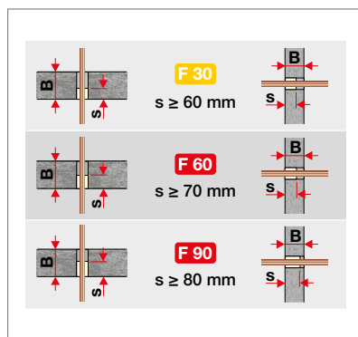
Abb. 196: Mindestabschottungsdicken bei Decke und Wand (deutsche Leitungsanlagen-Richtlinie)
