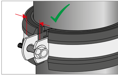
Abb. 272: Gleitschelle: empfohlene Montage
