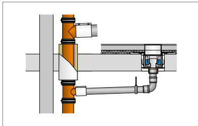
Abb. 230: Viega Advantix R 120 Bodenablauf und Rohrdurchführung – Mischinstallation
