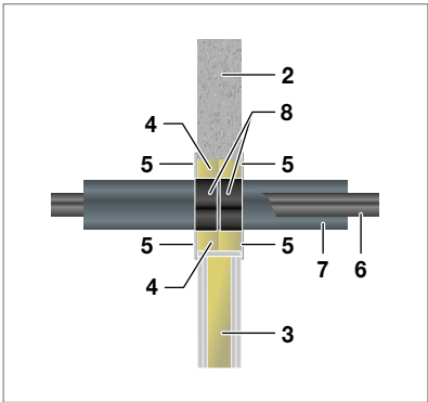
Abb. 213: Weichschott in der Massivwand und leichte Trennwand mit Viega Rohrleitungssystem Kunststoff
