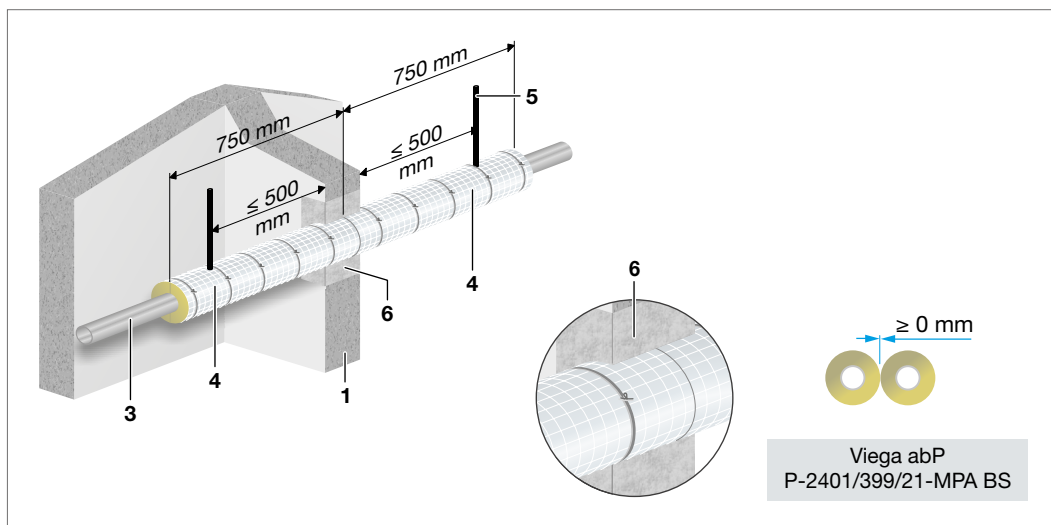
Abb. 163: Prestabo/Presstabo PP – Einbau in Massivwand
