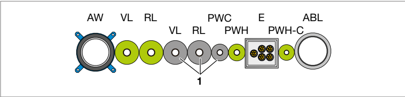
Abb. 200: optimierter Schacht durch Viega Brandschutzsystem mit Kühl- und Kälteleitungen im Schacht
