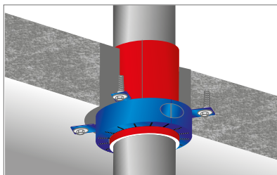
Abb. 266: Brennbare Abwasserrohr, durchgeführte PE-Dämmung, Brandschutzmanschette mit der Decke verschraubt, siehe Viega Verwendbarkeitsnachweis P-2400/003/15-MPA BS vom 07.03.2016
