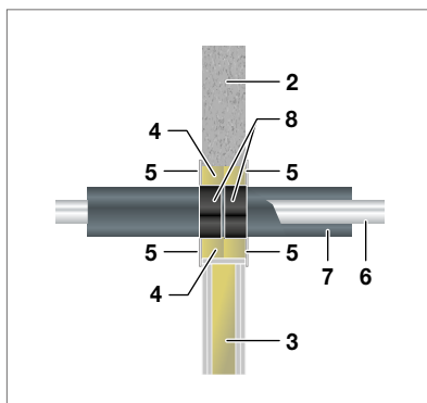
Abb. 211: Weichschott in der Massivwand und leichte Trennwand mit Viega Rohrleitungssystem Metall
