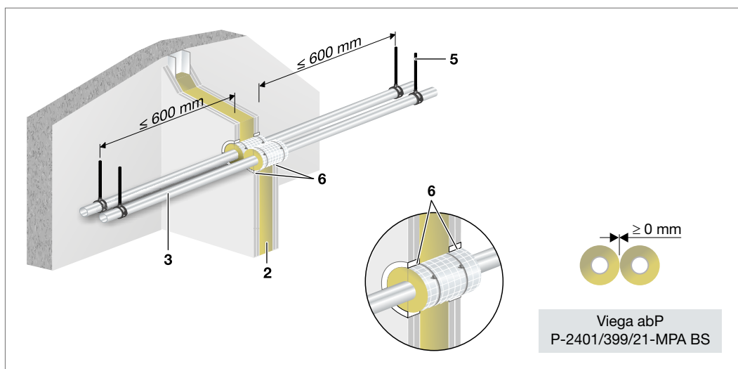
Abb. 172: Raxinox – Einbau in leichte Trennwand
