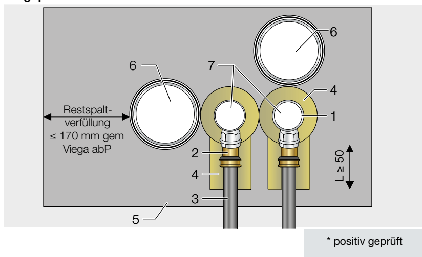
Abb. 137: Abschottung nach aBG Z-19.53-2714
