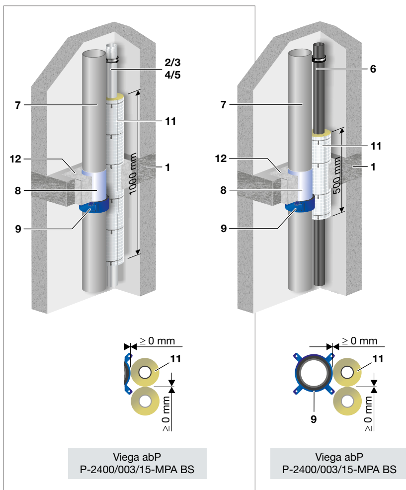
Abb. 131: Beispiele – Brandschutzmanschette Doyma mit allen Rohrtypen, nach Tab. 53
