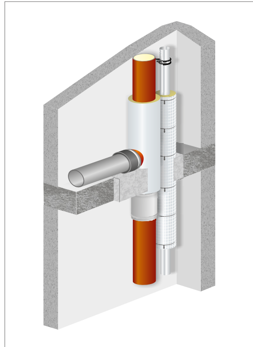
Abb. 271: Beispiel – Saint Gobain HES SVB Steckverbinder Einbau nach Z-19.17-2130, Anlage 4, Strang \leq 160 mm
