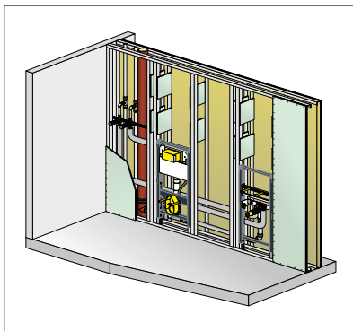
Abb. 293: Viega Prevista Dry – Inwandmontage
