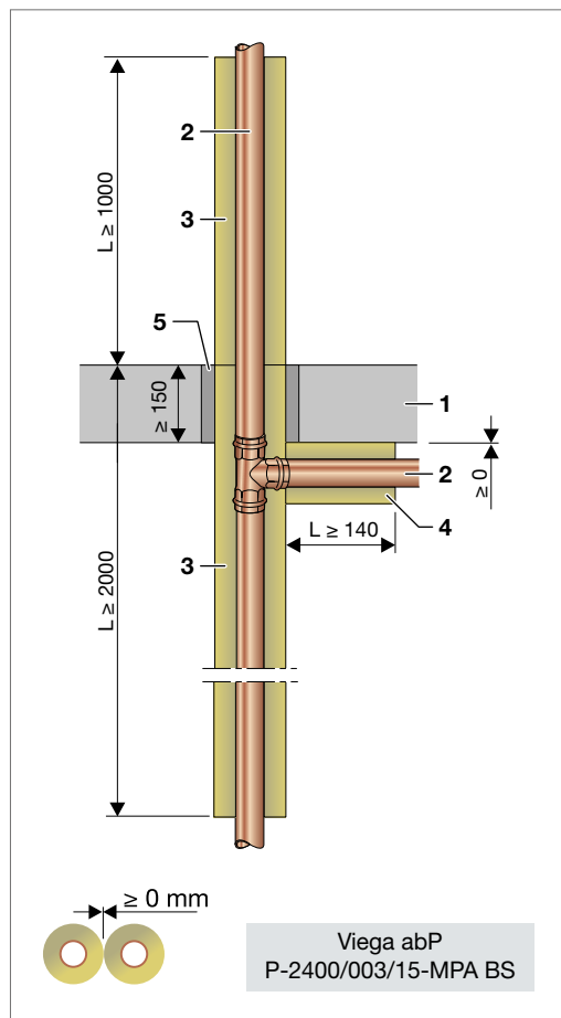
Abb. 66: Etagenbindung mit Profipress – unterhalb der Decke
