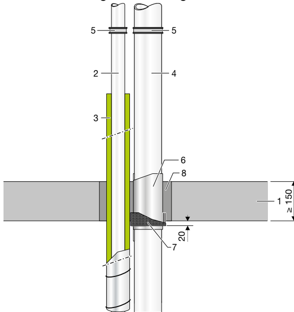
Abb. 135: Abstände zwischen Abschottungen nach dieser abG und Abschottungen nach abP Nr. P-2400/003/15-MPA BS
