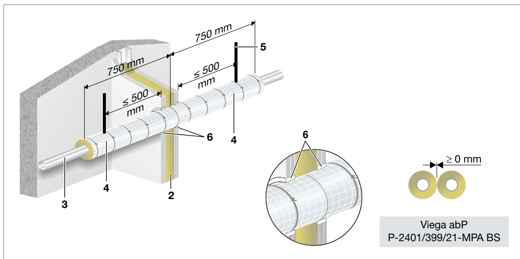
Abb. 158: Sanpress/Sanpress Inox/Sanpress Inox mit Smartloop Inliner-Zirkulation – Einbau in leichte Trennwand
