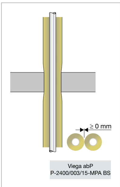
Abb. 141: Dämmung in Durchführung \leq 33\% komprimiert
