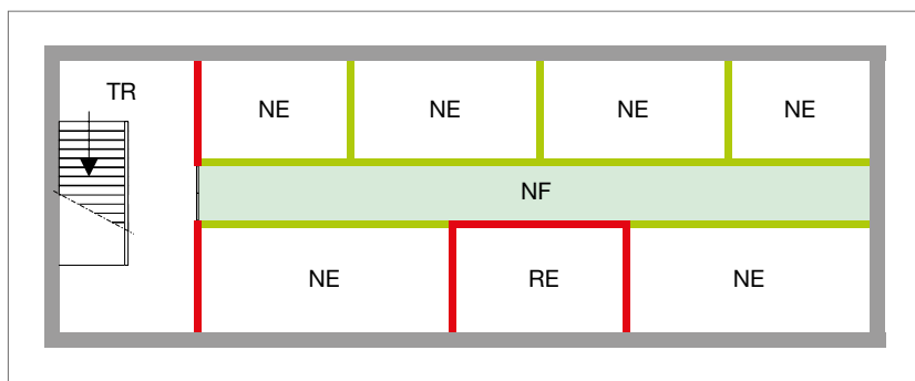
Abb. 214: Notwendiger Flur und Trennwände nach Musterbauordnung — MBO
