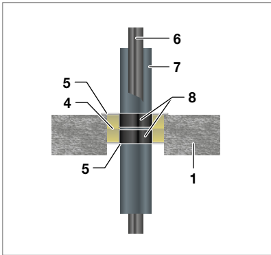
Abb. 212: Weichschott in der Massivdecke mit Viega Rohrleitungssystem Kunststoff
