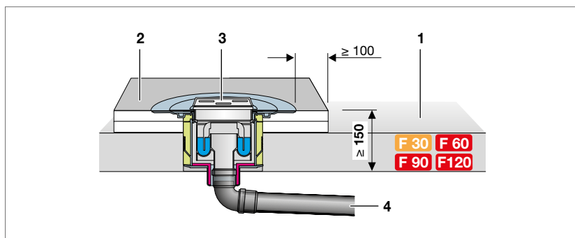
Abb. 240: Bodenablauf – Aufdoppelung \geq 100 mm umlaufend
