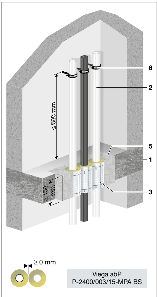
Abb. 110: Raxofix/Sanfix Fosta, d \leq 32 \text{ mm}
