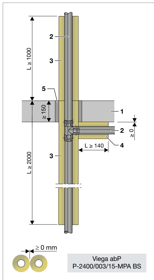
Abb. 103: Etagenansbindung mit Megapress – unterhalb der Decke
