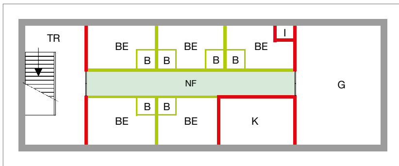
Abb. 187: Trennwände Beherbergungsstättenverordnung – MBeVO
