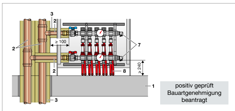
Abb. 186: Fußbodenheizung mit Viega Bauartgenehmigung, Viega Fonterra ( \leq DN25) Anschluss mit Viega Metallrohrsystem
