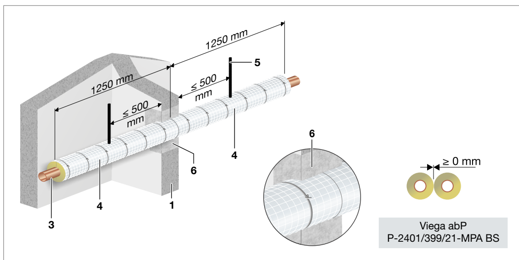
Abb. 155: Profipress/Profipress mit Smartloop Inliner-Zirkulation – Einbau in Massivwand
