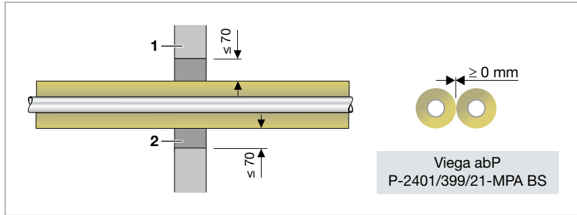
Abb. 181: Verschluss mit Mörtel
