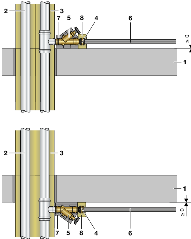
Abb. 42: Viega Easytop-Ventil/Rückflussverhinderer/Kugelhahn, positiv geprüft
