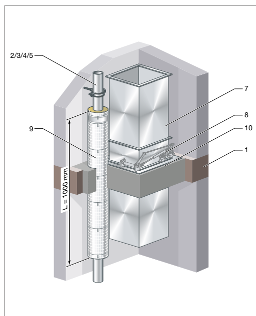
Abb. 144: Brandschutzklappen/EN1366-2
