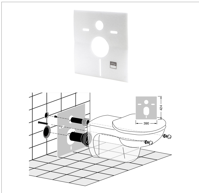
Abb. 303: WC-Schalldämmplatten
