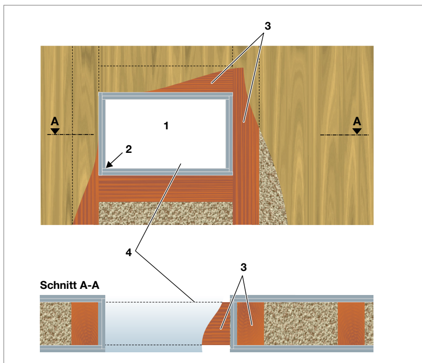
Abb. 154: Öffnungen in Holzbalkendecken mit Brandschutzbekleidung nach Abschnitt 3.2
