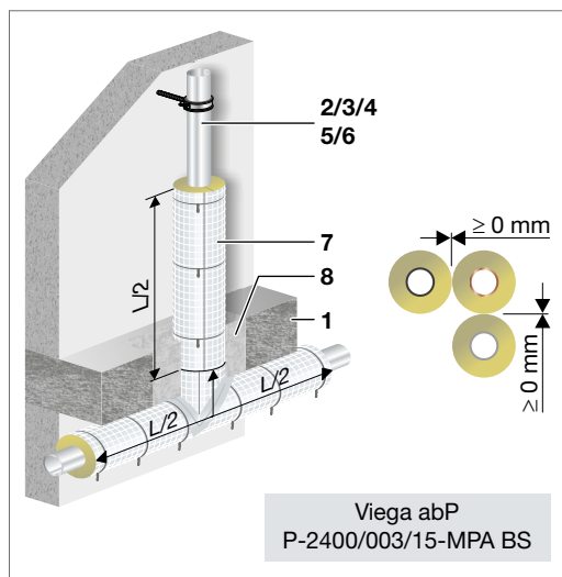
Abb. 120: Einbauvariante T-Stück
