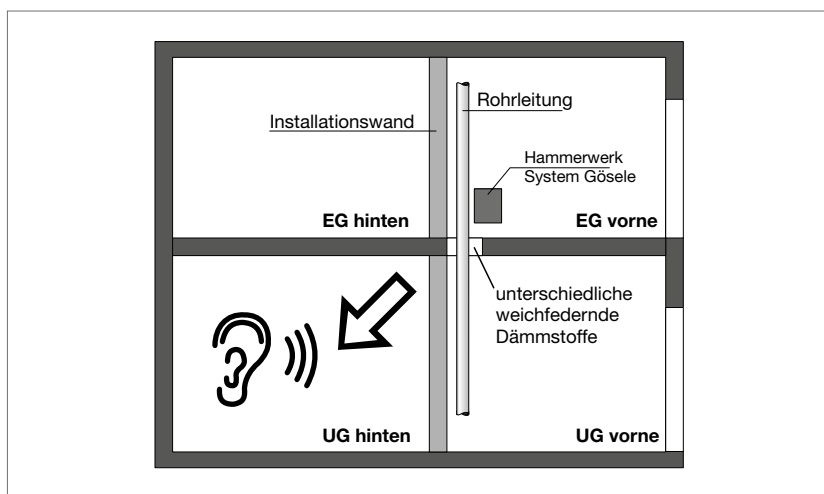
Abb. 265: Schnittzeichnung des Installationsprüfstands im Fraunhofer-Institut für Bauphysik. Der Prüfstand besteht aus je zwei übereinanderliegenden Räumen im Erd- und Untergeschoss (EG und UG), sodass in Verbindung mit Dach- und Kellergeschoss (DG und KG) auch über mehrere Stockwerke reichende Installation, wie z. B. Abwassersysteme, geprüft werden können.
