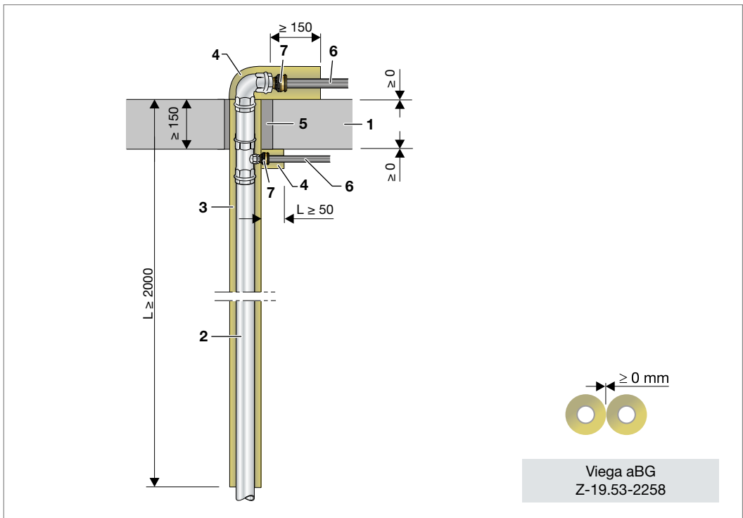
Abb. 83: Etagenbindung/oberstes Geschoss mit Temponox und Übergang auf Raxofix/Sanfix Fosta
