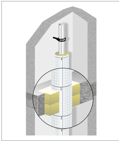
Abb. 202: Dämmung durch Weichschott hindurchgeführt – Decke
