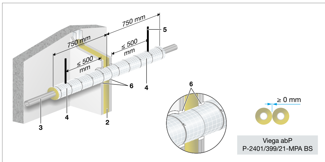
Abb. 164: Prestabo/Prestabo PP-ummantelt – Einbau in leichte Trennwand
