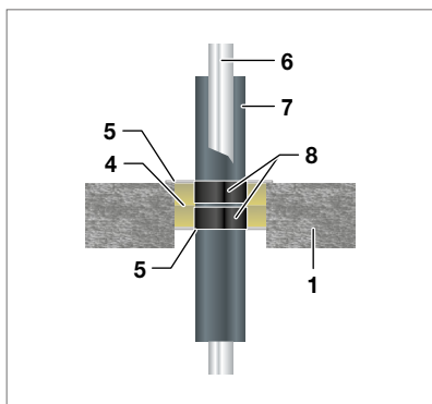
Abb. 210: Weichschott in der Massivdecke mit Viega Rohrleitungssystem Metall
