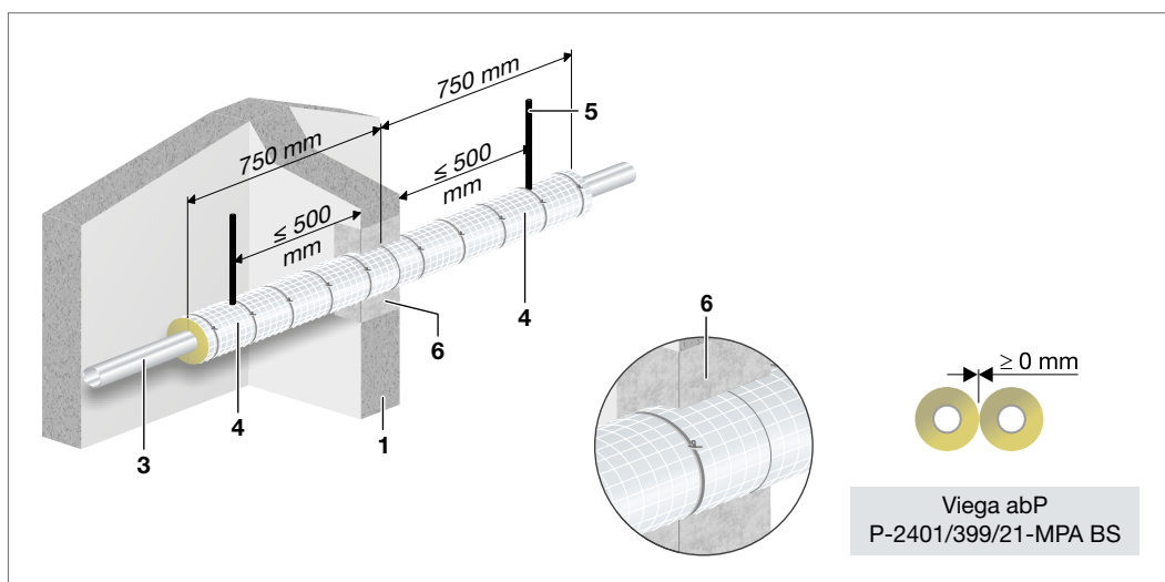
Abb. 159: Temponox – Einbau in Massivwand
