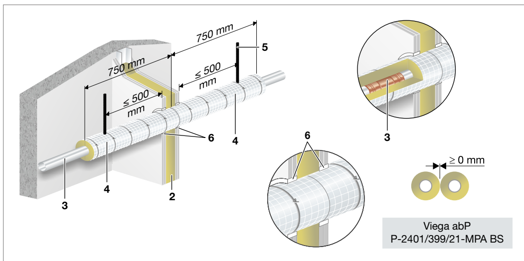
Abb. 162: Temponox in Verbindung mit Profipress Verbindern – Einbau in leichte Trennwand
