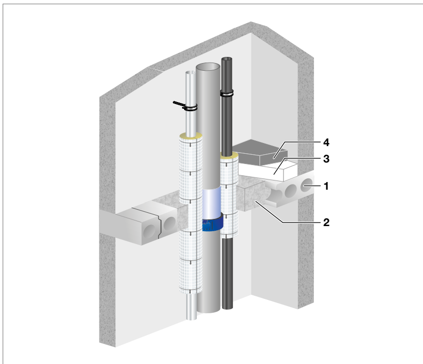
Abb. 150: Stahlbeton- und Spannbetonplatten aus Normalbeton mit Hohlräumen F 90-Konstruktion
