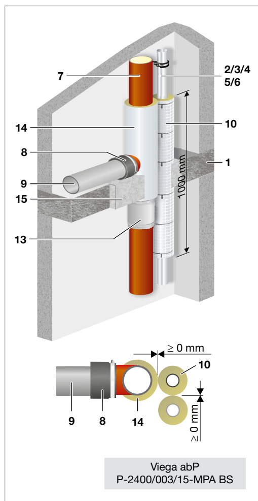
Abb. 126: Beispiel – Saint Gobain HES SVB Steckverbinder Einbau nach Z-19.17-2130, Anlage 4, Strang ≤ 160 mm
