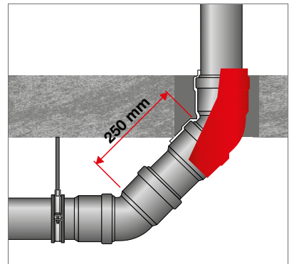
Abb. 275: Umlenkung am Fallstrang, Leitungslänge > 22 m mit Beruhigungs- strecke 250 mm
