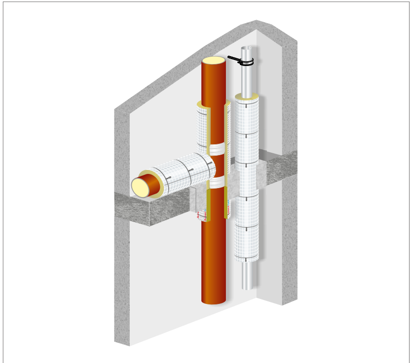
Abb. 268: Brandschutzsystem für Guss/SML-Leitungen mit formstabiler Brandschutzschale (Rockwool Conlit 150 U)
