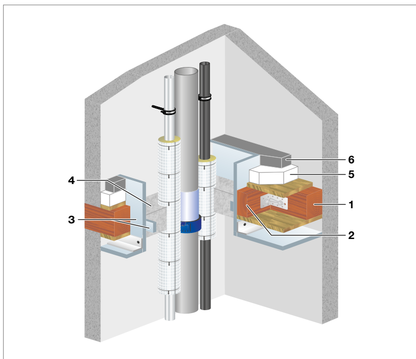
Abb. 148: Holzbalkendecke mit Unterdecke F 90-Konstruktion
