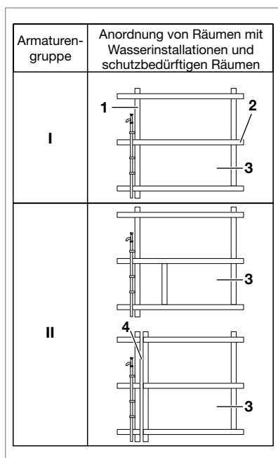
Abb. 249: Anordnung von Räumen mit Wasserinstallationen und schutzbedürftigen Räumen (Auszug aus DIN 4109-2018-01)
