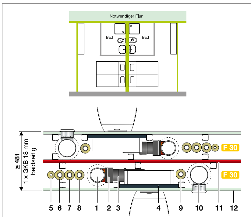
Abb. 228: F 30 Leichte Trennwand mit beidseitiger Wandbelegung
