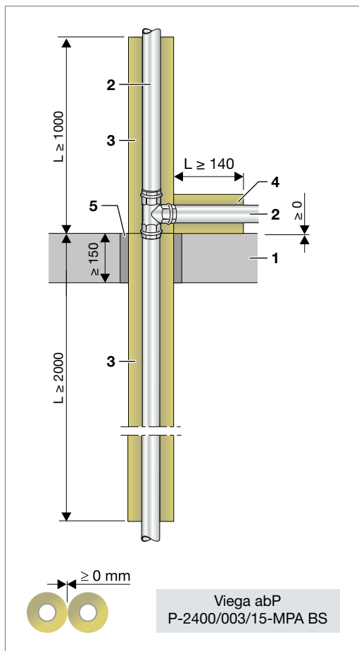
Abb. 81: Etagenansbindung mit Temponox – oberhalb der Decke
