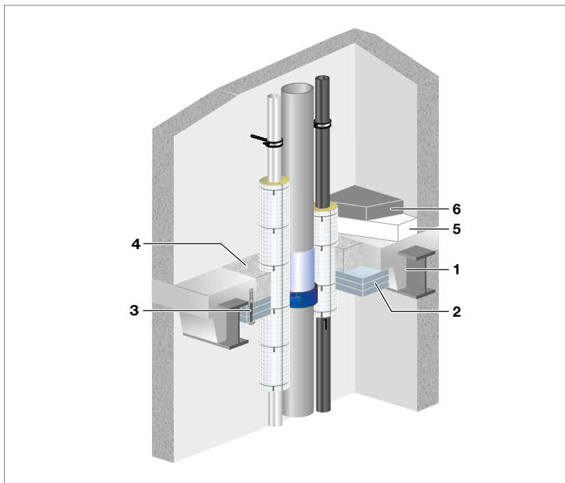
Abb. 152: Stahlbetondecke in Verbindung mit eingebetteten Stahlträgern aus Normalbeton bzw. Leichtbeton mit geschlossenem Gefüge nach DIN 4102-1 und -2 ohne Zwischenbauteile – F 30-, F 60-, F 90-Konstruktion
