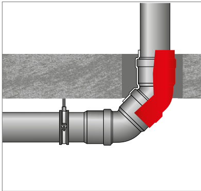
Abb. 274: Umlenkung am Fallstrang 2x45°-Bogen
