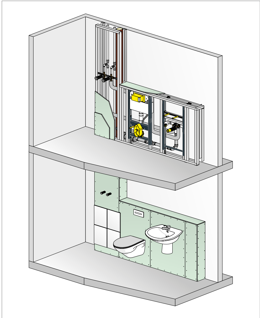
Abb. 297: Vorwand-Installation mit Viegä Prevista Dry vor Massivwand (Darstellung beispielhaft)
