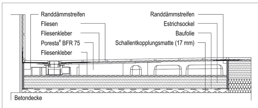
Abb. 286: Systemaufbau einer bodengleichen Dusche
