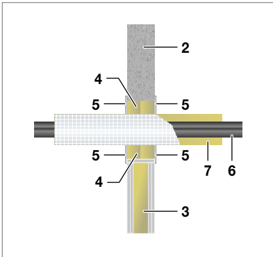
Abb. 209: Weichschott in der Massivwand und leichte Trennwand mit Viega Rohrleitungssystem Kunststoff
