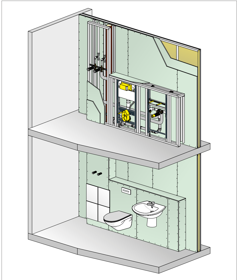
Abb. 299: Vorwand-Installation mit Viega Prevista Dry vor leichter Trennwand (Darstellung beispielhaft)
