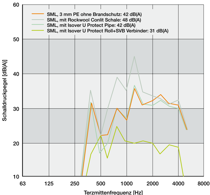
Abb. 269: Summenschallpegel im UG hinten
