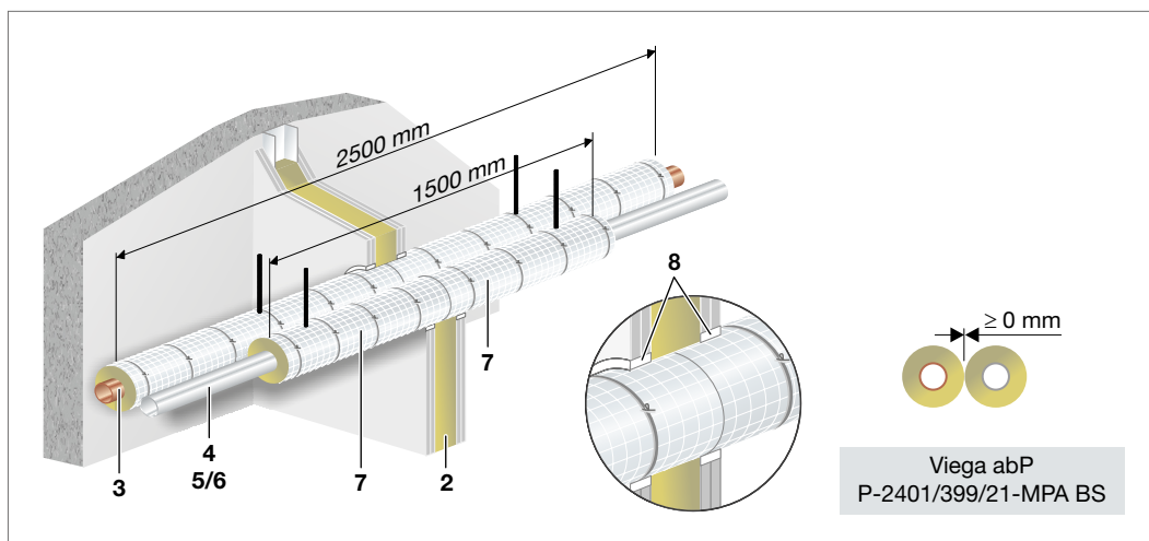
Abb. 174: Einbau in leichte Trennwand
