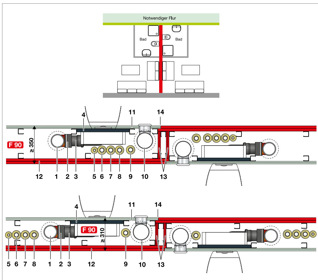
Abb. 227: F 90 Leichte Trennwand mit beidseitiger Wandbelegung
