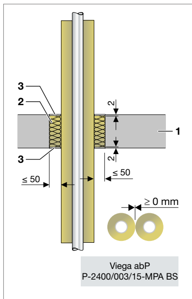
Abb. 140: Viega Brandschutz-Kitt/lose Wolle
