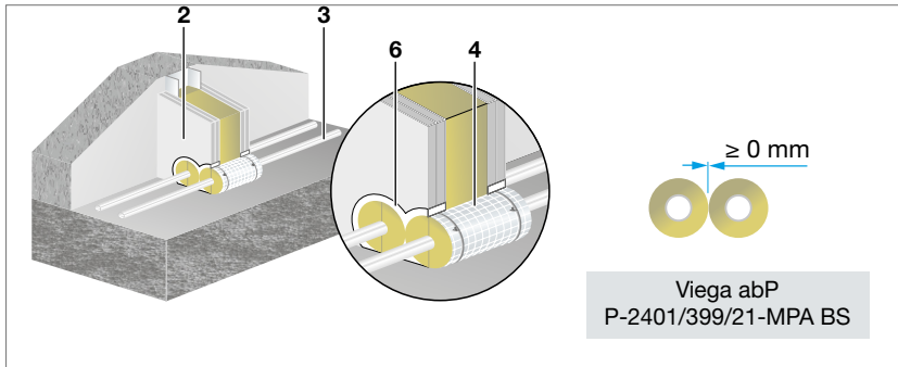
Abb. 191: Wanddurchführung mit Sanfix Fosta/Raxofix, d = 16 mm, durch leichte Trennwand, R 30/R 60/R 90
