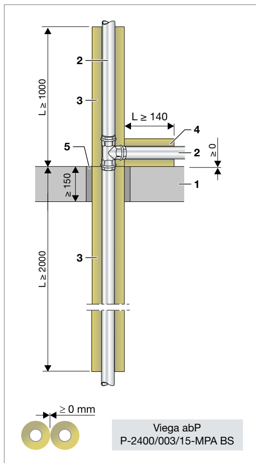
Abb. 75: Etagenansbindung mit Sanpress/Sanpress Inox – oberhalb der Decke
