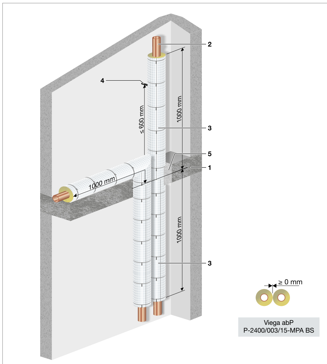
Abb. 59: Profipress/Profipress mit Smartloop Inliner-Zirkulation
