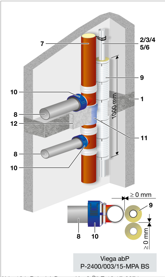
Abb. 124: Beispiel-Doyma Konfix Pro Z-19.17-2074
