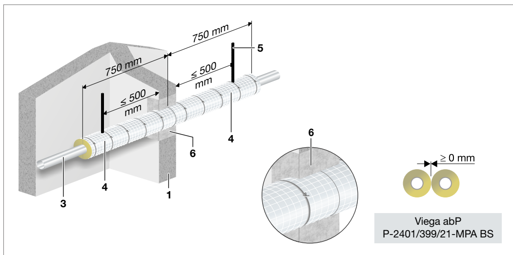
Abb. 157: Sanpress/Sanpress Inox/Sanpress Inox mit Smartloop Inliner-Zirkulation – Einbau in Massivwand
