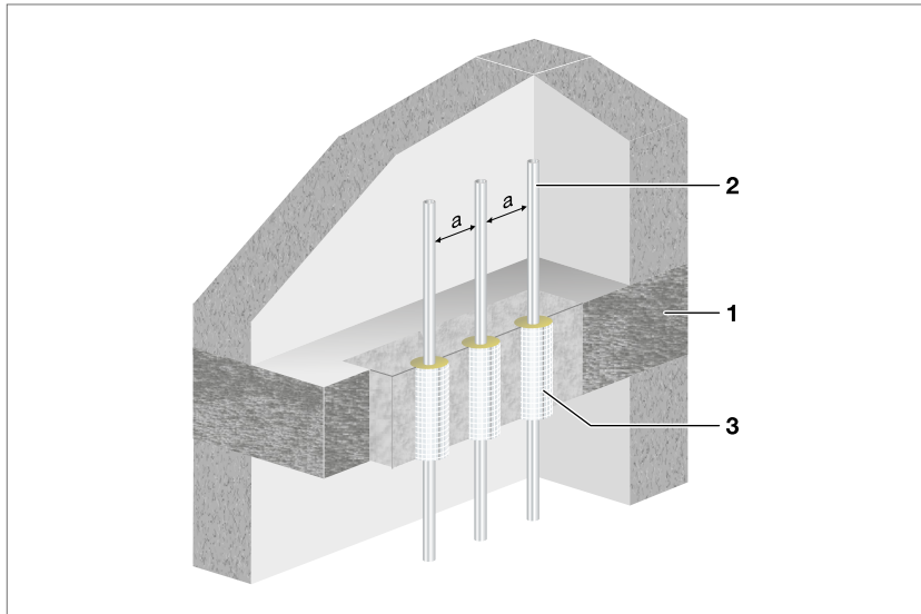
Abb. 194: Deckendurchführung Fonterra Rohre/Raxofix/Sanfix Fosta nach LAR
