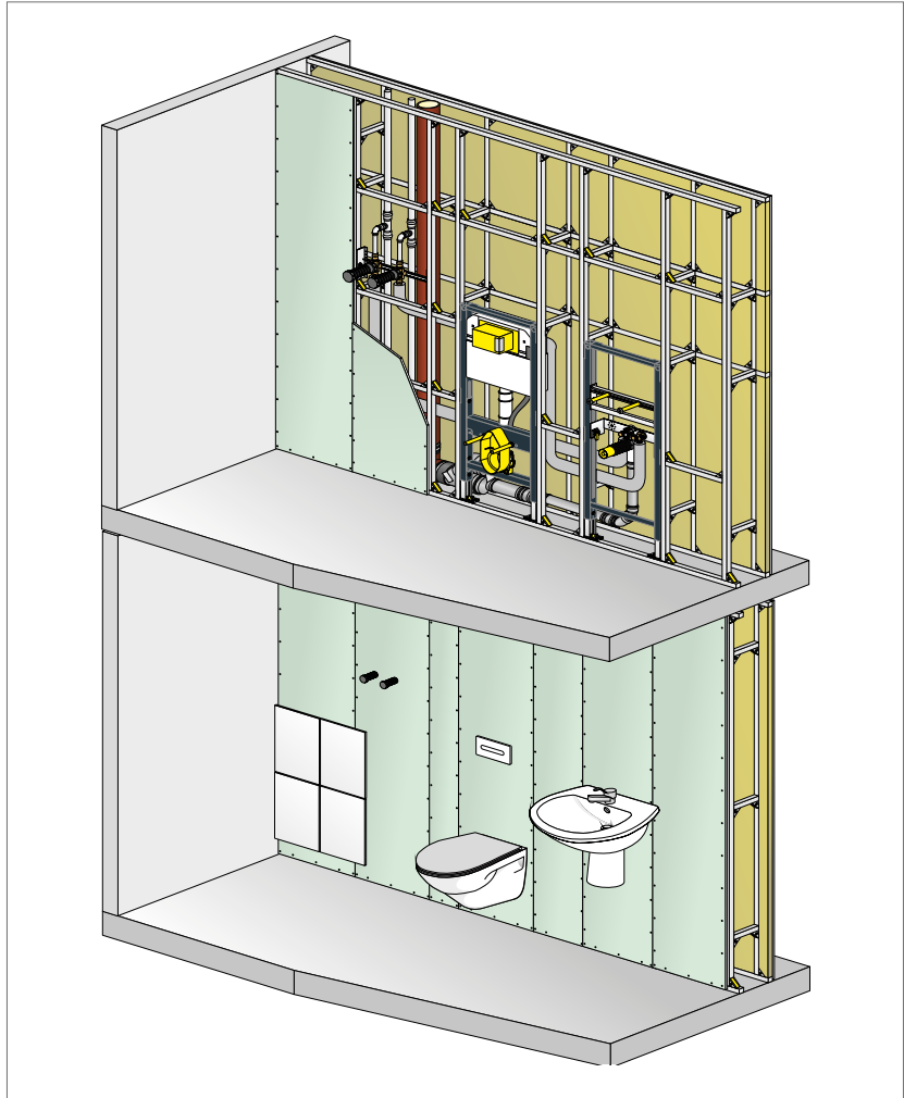
Abb. 295: Installationswand mit Prevista Dry Plus (Darstellung beispielhaft)
