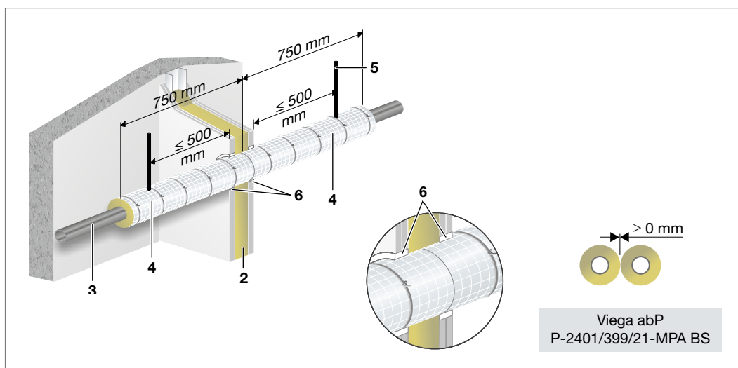
Abb. 166: Megapress – Einbau in leichte Trennwand
