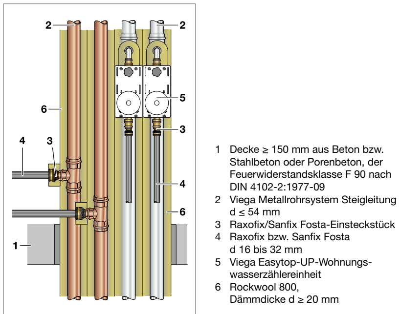
Abb. 25: Beispiel Mischinstallation im Wohnungsbau
