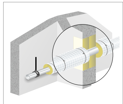
Abb. 205: Unterbrochene Dämmung – Wand
