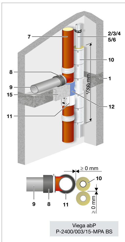
Abb. 125: Beispiel – Düker BSV 90, Z-19.17-1893
