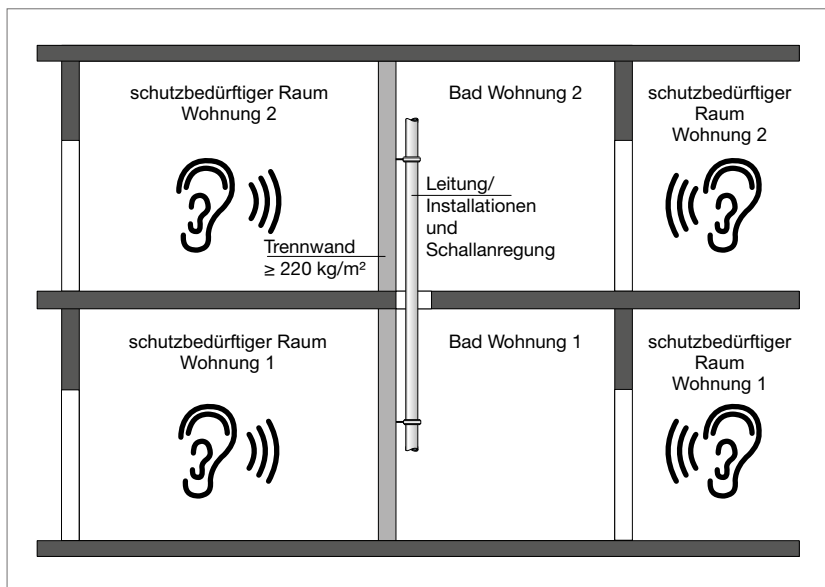
Abb. 250: Schallschutz im eigenen und fremden Wohnbereich nach VDI 4100
