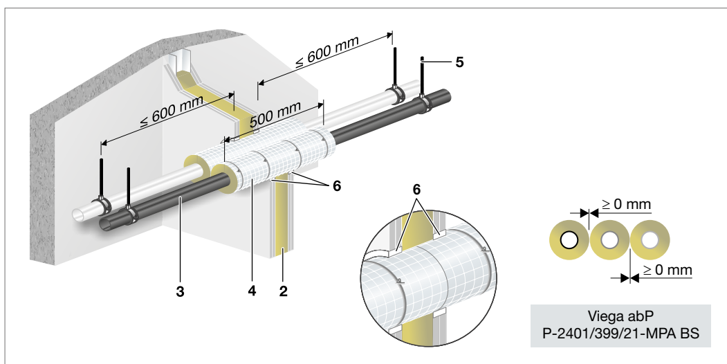
Abb. 168: Raxofix/Sanfix Fosta, d 16 - 63 mm – Einbau in leichte Trennwand
