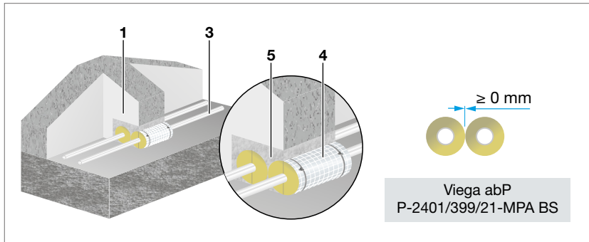
Abb. 190: Wanddurchführung mit Sanfix Fosta/Raxofix, d = 16 mm, durch Massivwand, R 30/R 60/R 90
