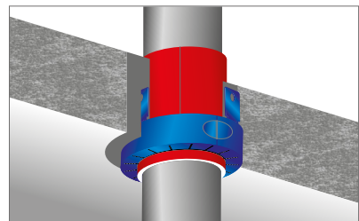
Abb. 264: Montagebeispiele von Brandschutzmanschette mit Schallschutzmatte aus PE, s = 5 mm (teilweise eingelassen)
