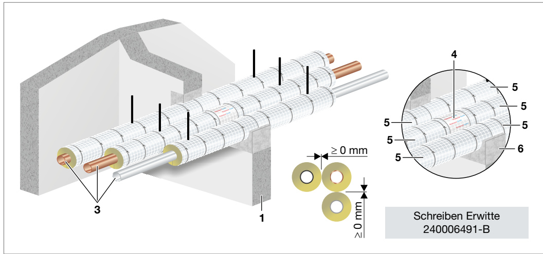
Abb. 175: Viega Metallrohrsysteme im Nullabstand Rockwool Conlit 150U ab P-3725/4130-MPA-BS – Massivwand
